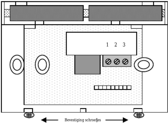
Tekening 1: Muur/Bodemplaat
